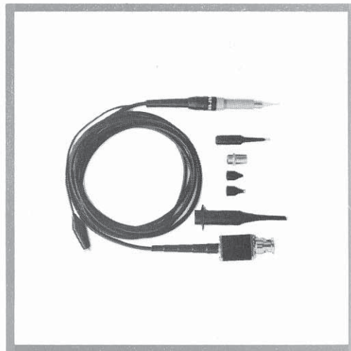
Oszilloskop-Tasterdivisor 100 : 1 HZ 37
