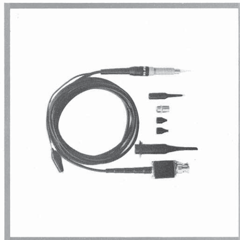
Oszilloskop-Tasterdivisor 10 : 1 HZ 38
